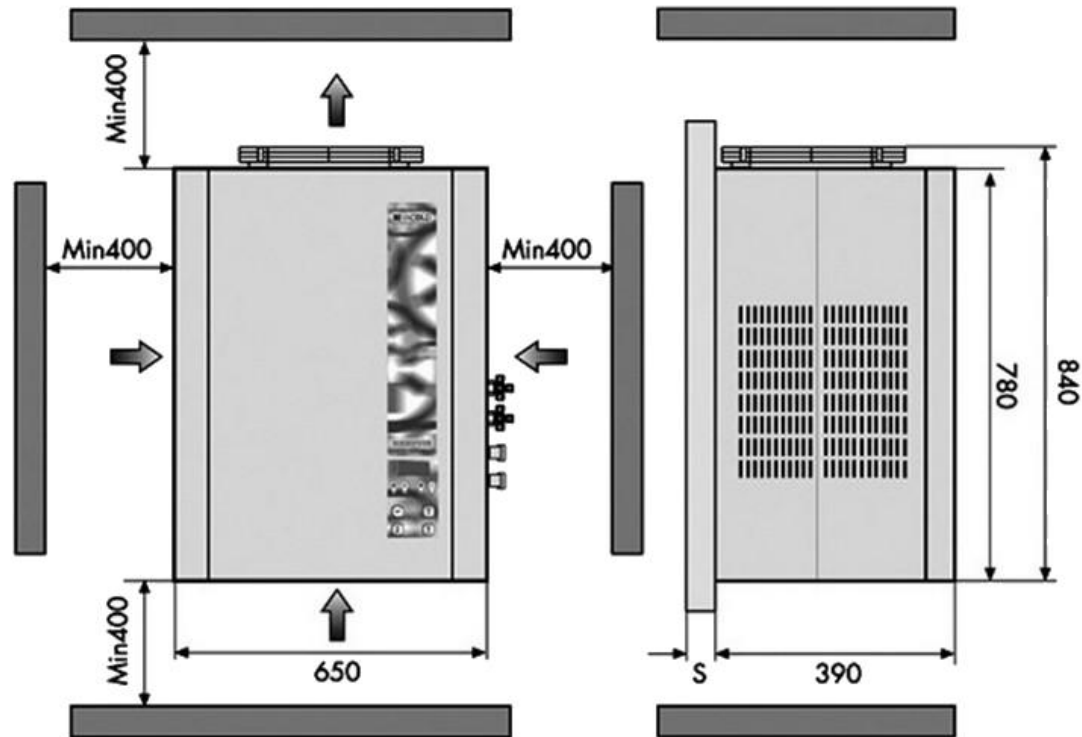
Vorderansicht
