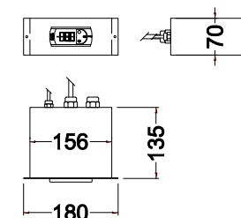
Elektronisches Thermostat
