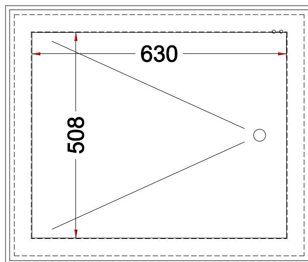
(Draufsicht)
