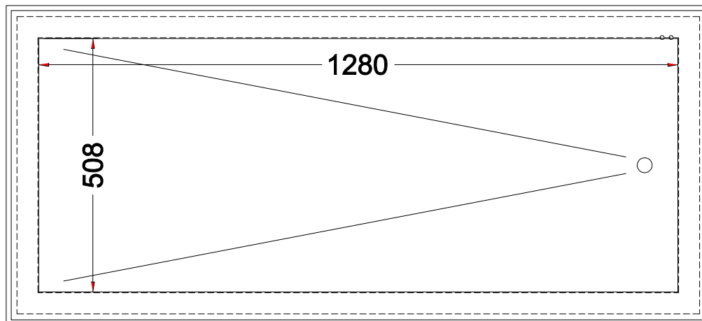
(Draufsicht)
