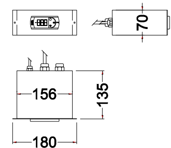
Elektronisches Thermostat
