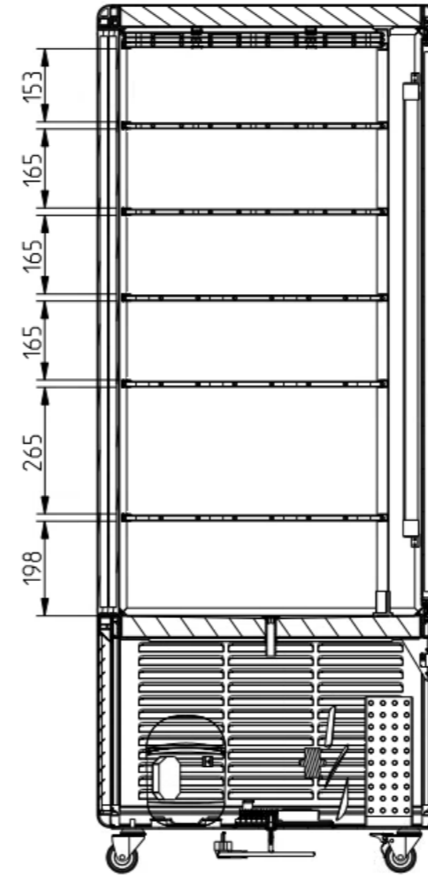
Seitenansicht
