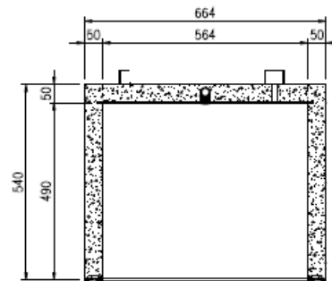
SEZIONE A-A
